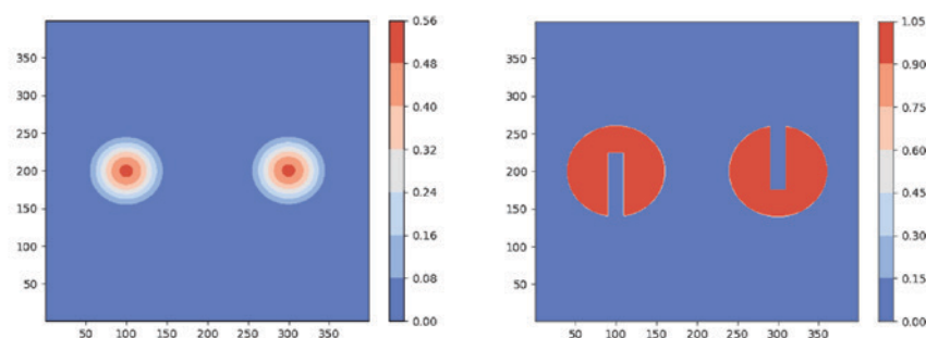
Рис 1. Начальное значение плотности льда с гладким профилем (слева), с разрывным профилем (справа).
