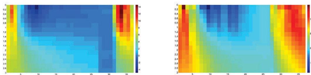
Рис. 1. Изменение температуры по глубине (по вертикали, метры) и по времени (по горизонтали, декады) на перевале Анзоб (Гиссарский хребет) за сезон наблюдений 2019-2020 года на северном и южном макросклоне.
