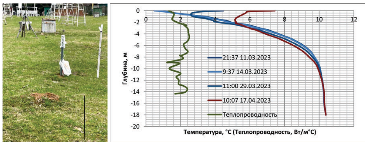
Рис. 1. Внешний вид скважины и изменение температуры по глубине (по вертикали метры, по горизонтали температура) на площадке МО МГУ в начале 2023 года.
