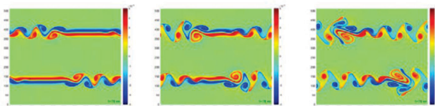
Рисунок 2. Поле относительной завихренности численного решения с локальным сгущением (128x128 и 256x256 точек, 10-12-15 суток).
