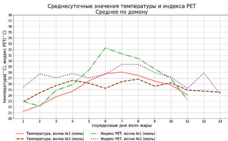
Рис. 1. Ход температуры и индекса PET за периоды волн жары.
